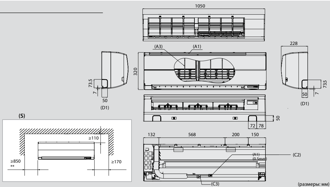
RBC-AMS41E
