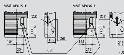
Положение труб фреоновой трассы
