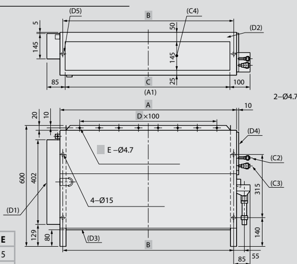
TCB-AX21E2 TCB-AX32E2
